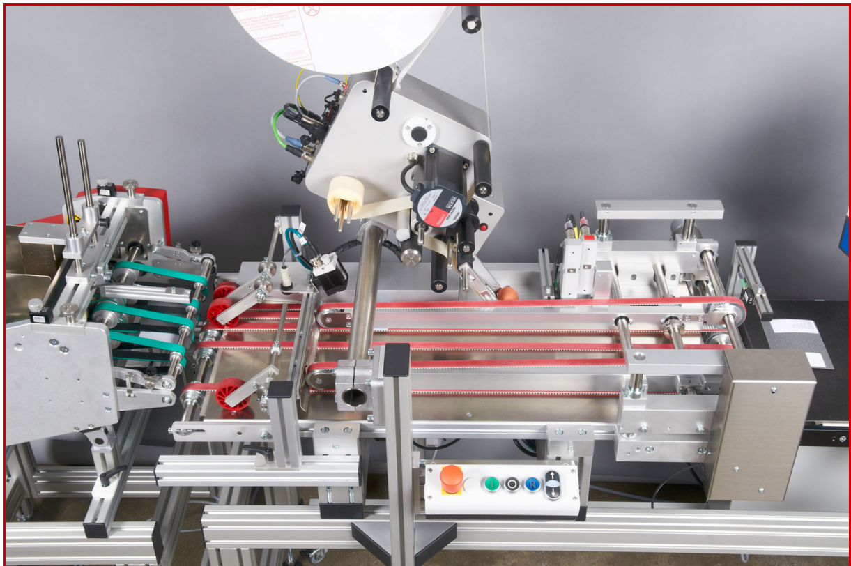
Transportsystem mit Kamera, Etikettierer und HP basierendem Ink-Jet-System
